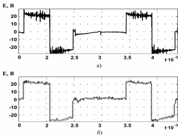
Рис. 5. Фазные ЭДС при работе ВРД на «естественной» механической характеристике: а) – расчет, б) – эксперимент.
