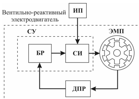
Рис. 1. Функциональная схема вентильно-реактивного двигателя
