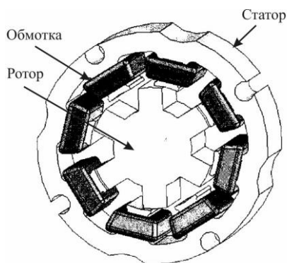
Рис. 4. Конструкция исследуемого четырехфазного электромеханического преобразователя
